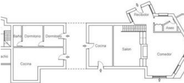
Planta Baja
