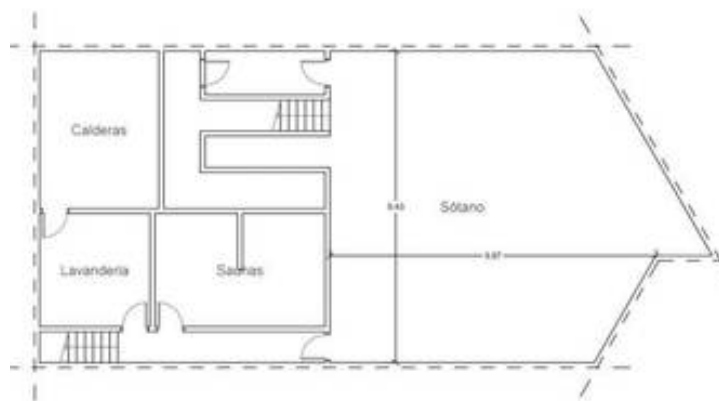
Planta Sótano
