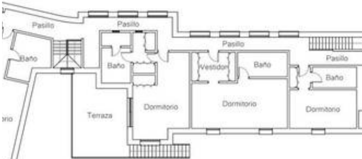
Planta Alta
