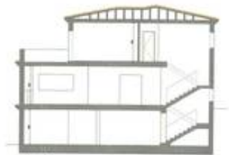
SECCION 1/1
